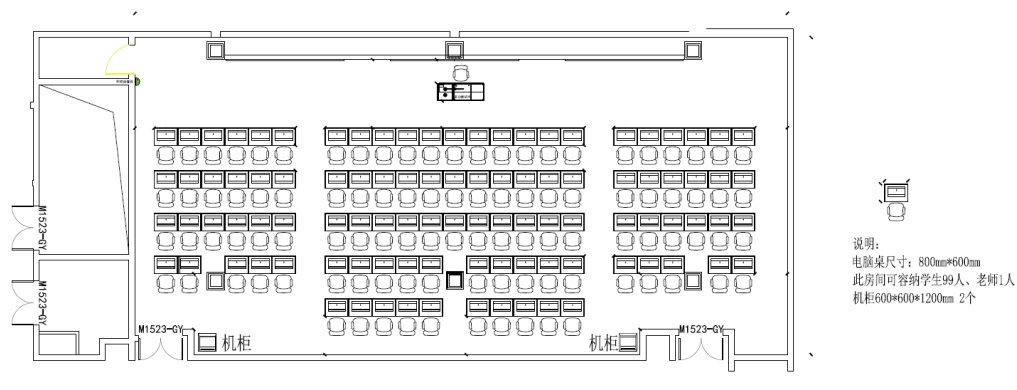
B1层多媒体教室（西区-B1-005）99人平面布局图 1:100
